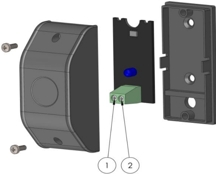
Şekil 3 Verici Emniyet Fotoseli Klemensleri
