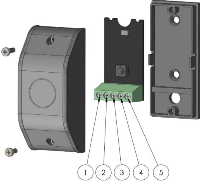
Şekil 2 Alıcı Emniyet Fotoseli Klemensleri
