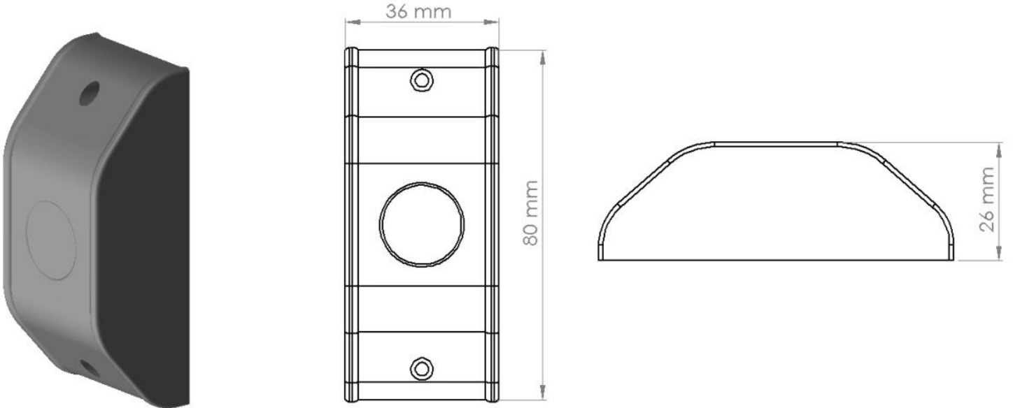
Şekil 1 Boyutlar
